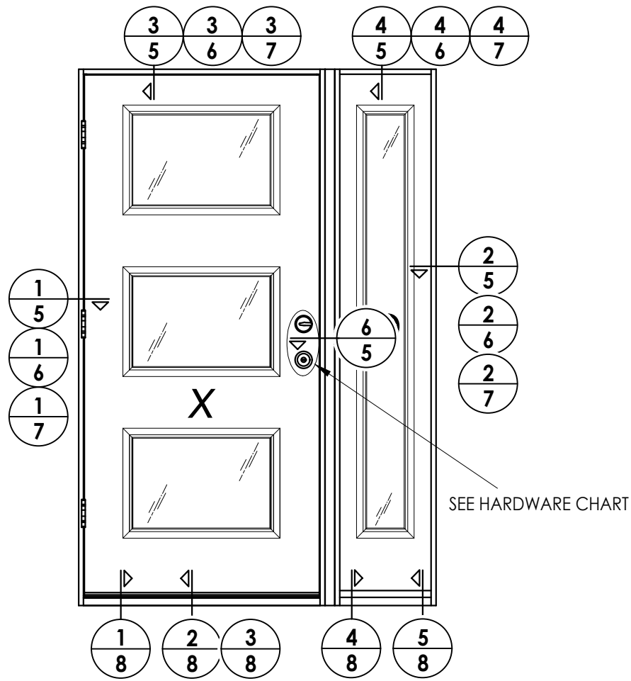
ELEVATION XO
