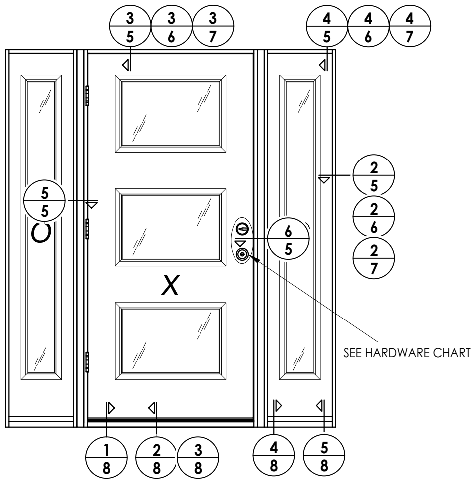
ELEVATION OXO
